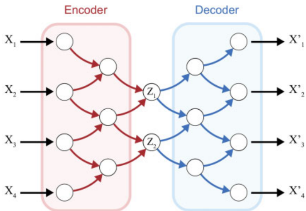
(a) Autoencoder
